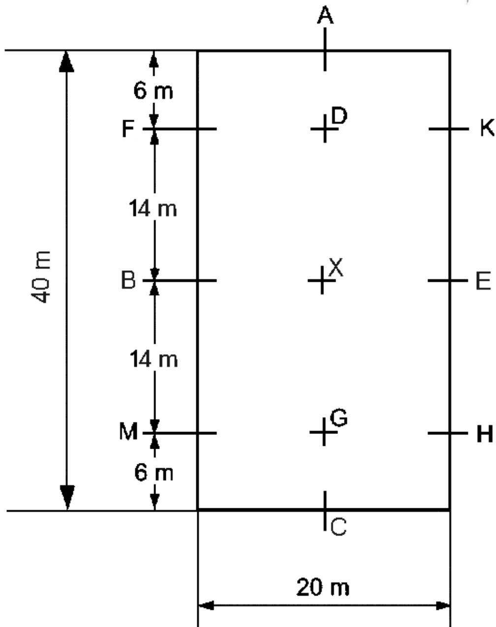
Schemat czworoboku 20 x 40
